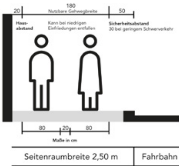
Abb. 15: Nutzare Gehwegbreite (Quelle: EFA, Bild 4)
