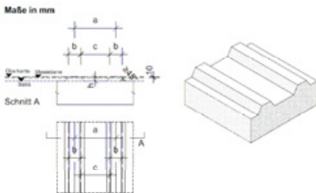
Abb. 29: Profil Rippenplatten (gemäß DIN 32984:2020-12)
