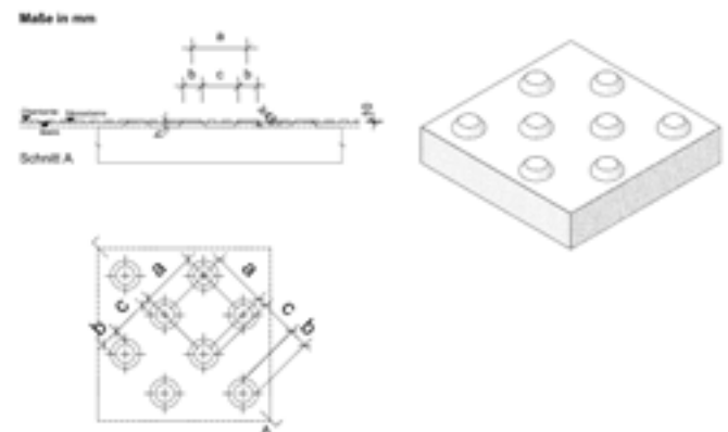
Abb. 30: Profil Noppenplatten (gemäß DIN 32984:2020-12)
